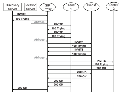
Bild 5 Aufruf einer Dienstekombination mit SIP
