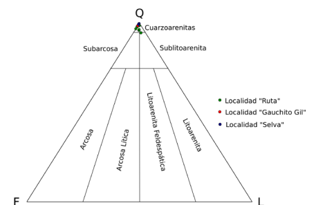
Figura 4. Clasificación petrográfica de las areniscas según Folk (1974). Q: cuarzo mono y policristalino (excluyendo chert); F: feldespatos; L: fragmentos líticos (ígneos, metamórficos y sedimentarios, incluyendo chert)
