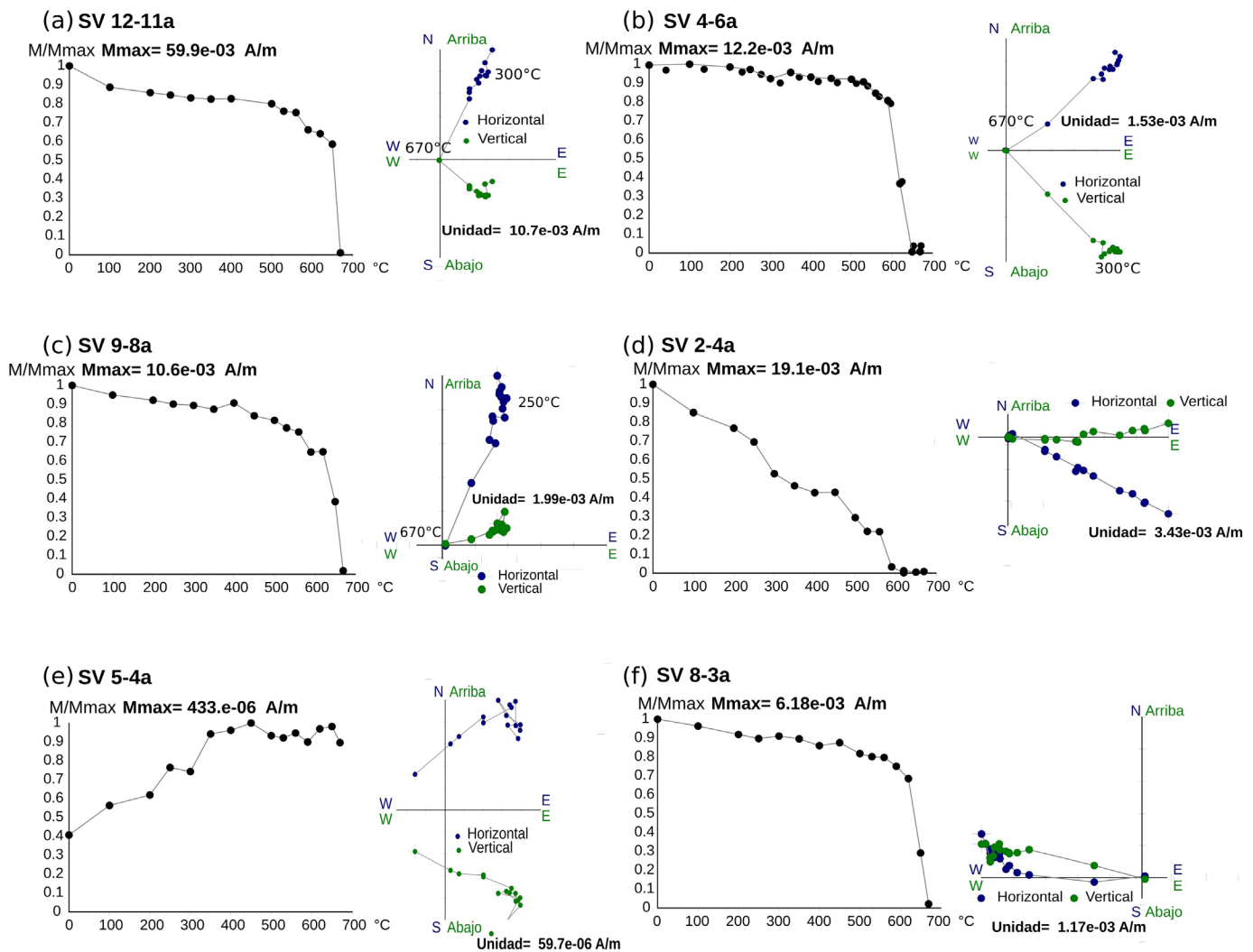
Figura 7. Diagramas de Zijderveld junto con su correspondiente curva de desmagnetización para los especímenes: a) SV 12-11a; b) SV 4-6a; c) SV 9-8a; d) SV 2-4a; e) SV 5-4a y f) SV 8-3a. Observar que la desmagnetización ocurre entre los 650 y los 670°C. Notar en: (c) la presencia de dos componentes, una hasta 250°C y otra, hasta 670°C; (d) el decaimiento más progresivo de la curva de desmagnetización en comparación los casos anteriores, lo que marca la existencia de un patrón distribuido de temperatura de bloqueo; (e) no se terminan de aislar las componentes, por lo cual se aplica posteriormente el método de círculos máximos; (f) espécimen de un sitio cuya componente característica tiene una polaridad opuesta.
